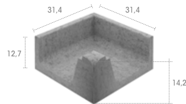
RS 933 Esquina Interior Inside corner Angle intérieur
