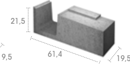
RS 916 Escalera abierta, esquina derecha Open built-in stairs, right corner Échelle ouverte, coin droit
