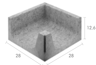
RS 943 Esquina Interior Inside corner Angle intérieur
