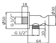
SOPORTE CON TOMA DE AGUA CILINDRICO BRASS SUPPORT WITH 1/2" CYLINDRIQUE WALL OUTLET SUPPORT CYLINDRIQUE AVEC PRISE D'EAU
